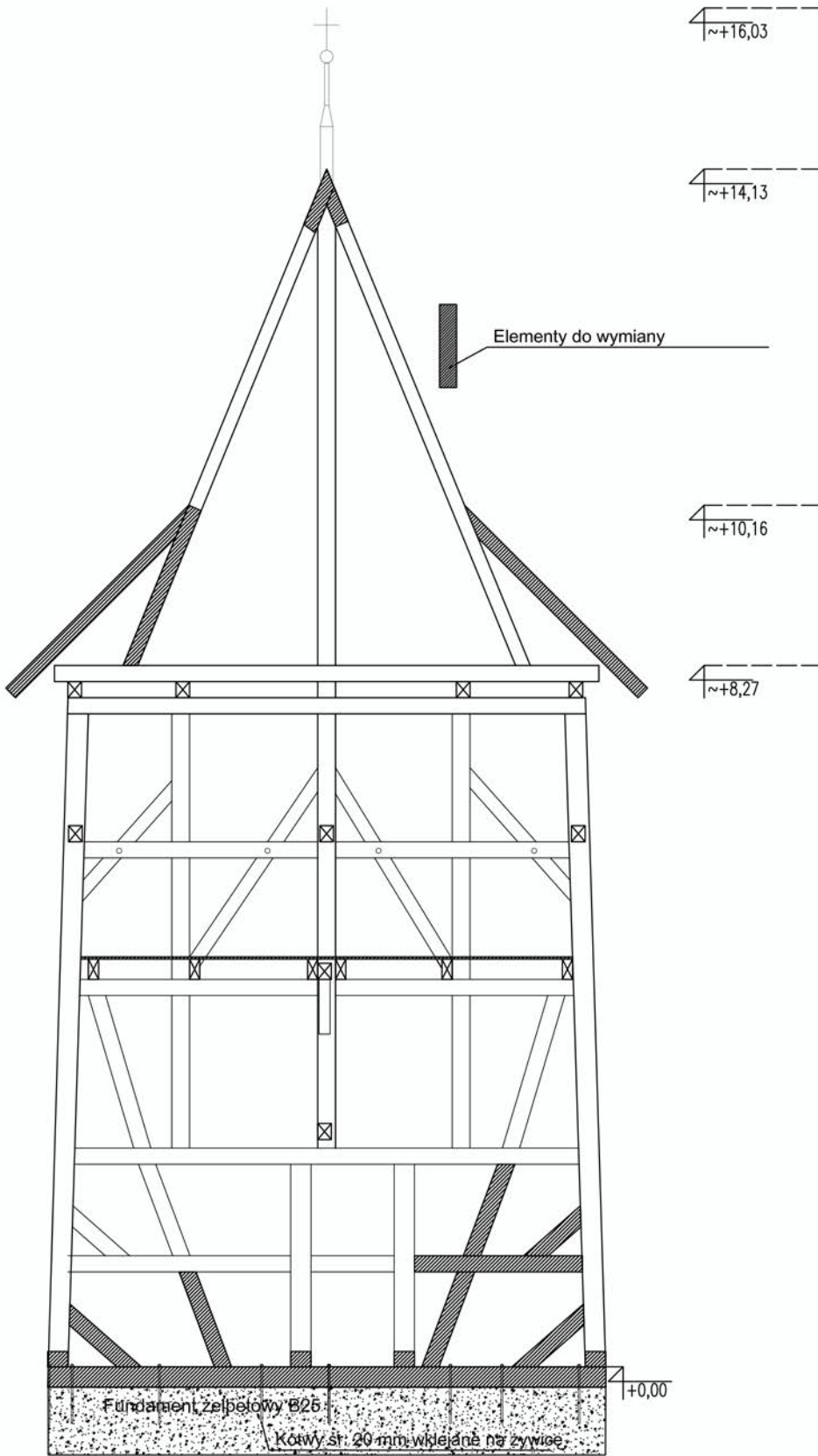
WIDOK KONSTRUKCJI ŚCIANY WSCHODNIEJ A0-A0
